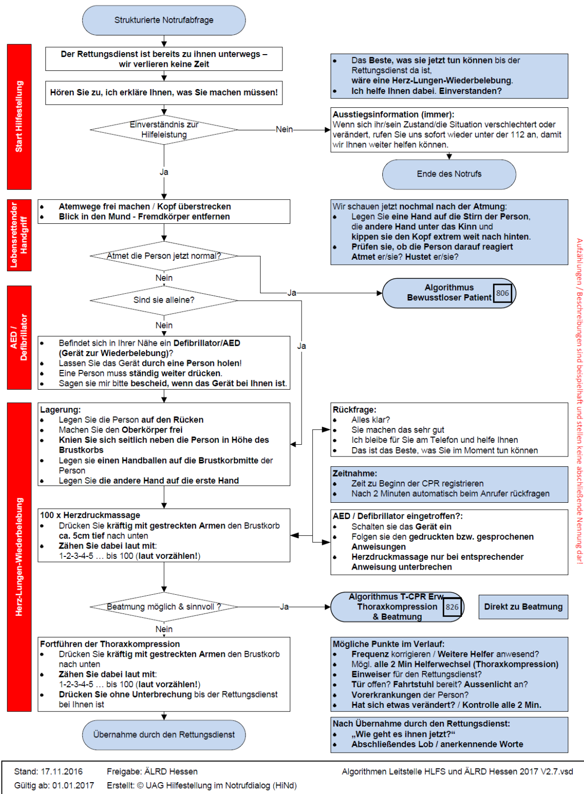
Abb. 5: Hessischer T-CPR-Algorithmus 2017
